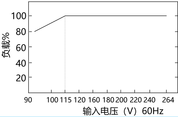
输入电压降额曲线图
