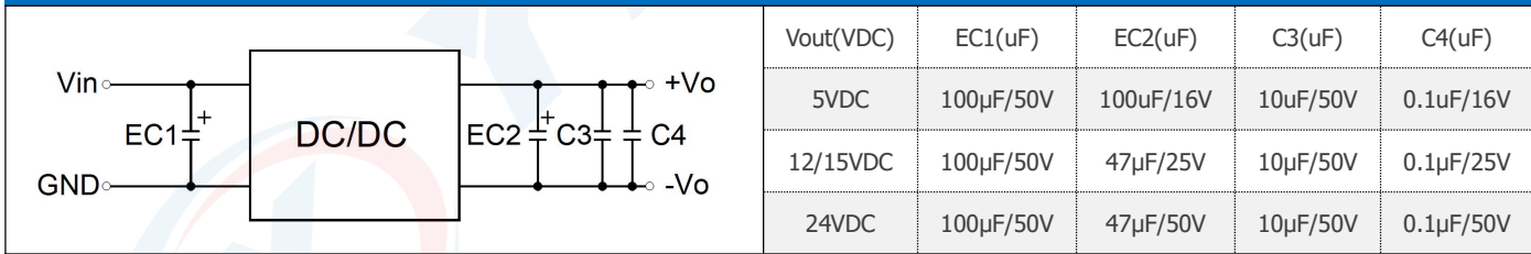
应用电路（图 2） 推荐容性负载值表
