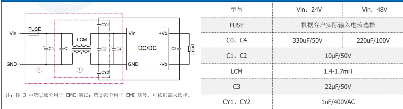
EMC 推荐电路（图 3） 推荐容性负载值表
