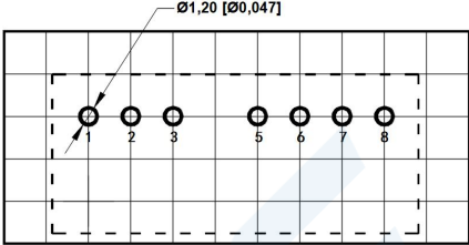
栅格距离尺寸为 2.54 x 2.54 mm
