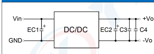
应用电路（图 2）
