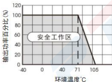
温度降额曲线图（图 1）
