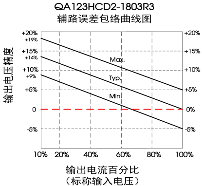
图 5 (辅路误差包络曲线)
