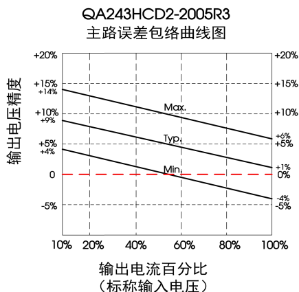
图 18 (主路误差包络曲线)
