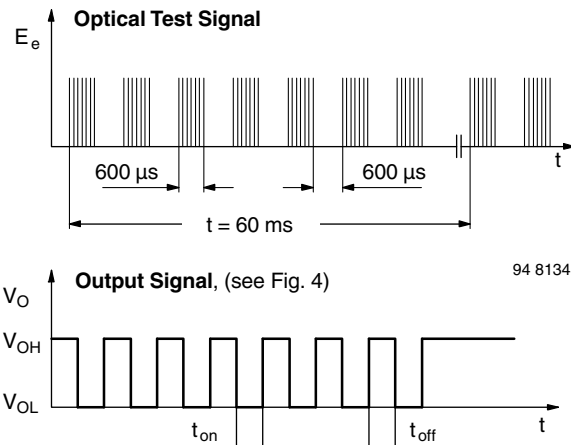
Fig. 3 - Output Function
