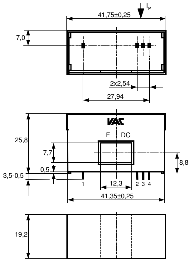
Maßbild Nr. 1
