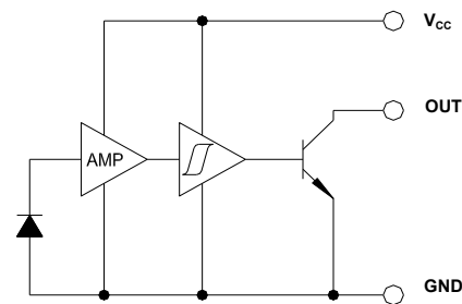
OPB761, OPB771 Buffered Open Collector
