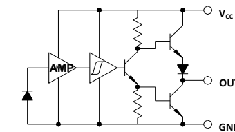
OPB717 Inverted Totem-Pole
