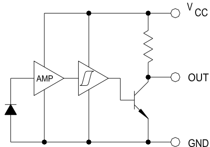
OPB687, OPB697 Inverted 10K Pull-Up
