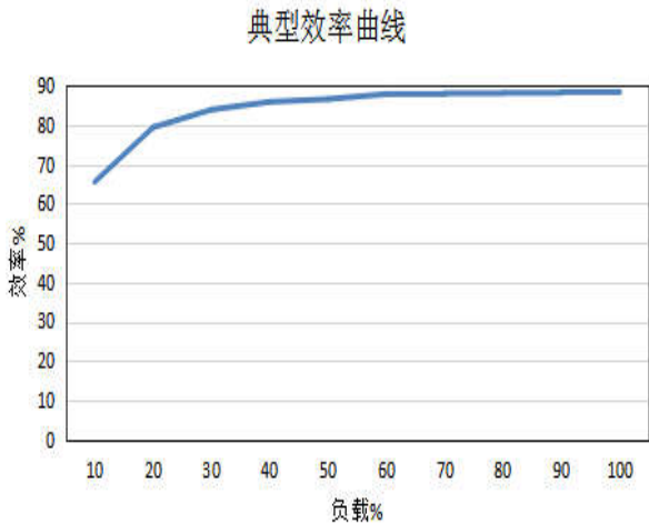
12V 输出时典型效率曲线图 图 5
