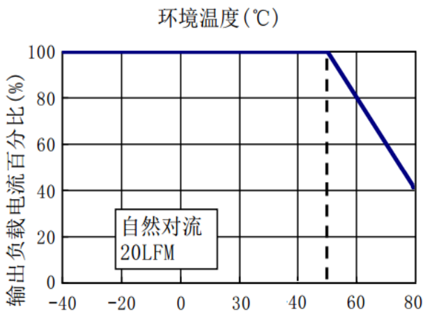
温度降额曲线 (°C)
