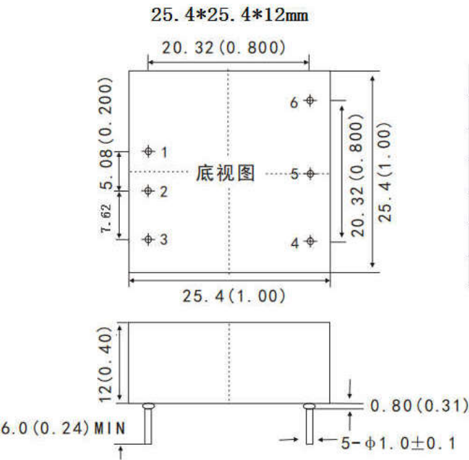
TDK20-XXSXXWHS 管脚定义及说明
