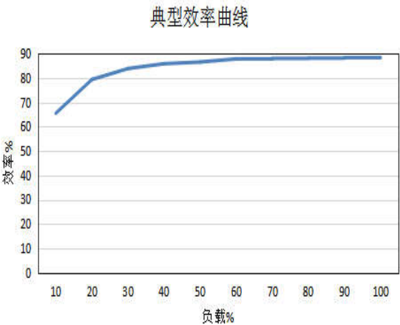
12V 输出时典型效率曲线图
