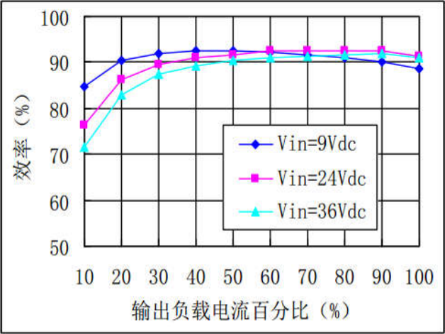
典型效率曲线图
