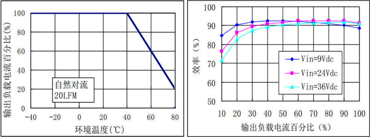
工作温度(°C) 图 4 12V 输出时典型效率曲线图 图 5
