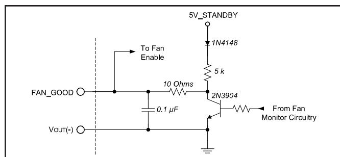
Figure A: Fan status output / Fan enable input interface circuitry.
