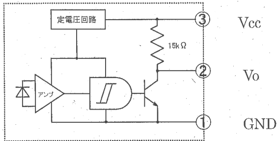
等価回路
