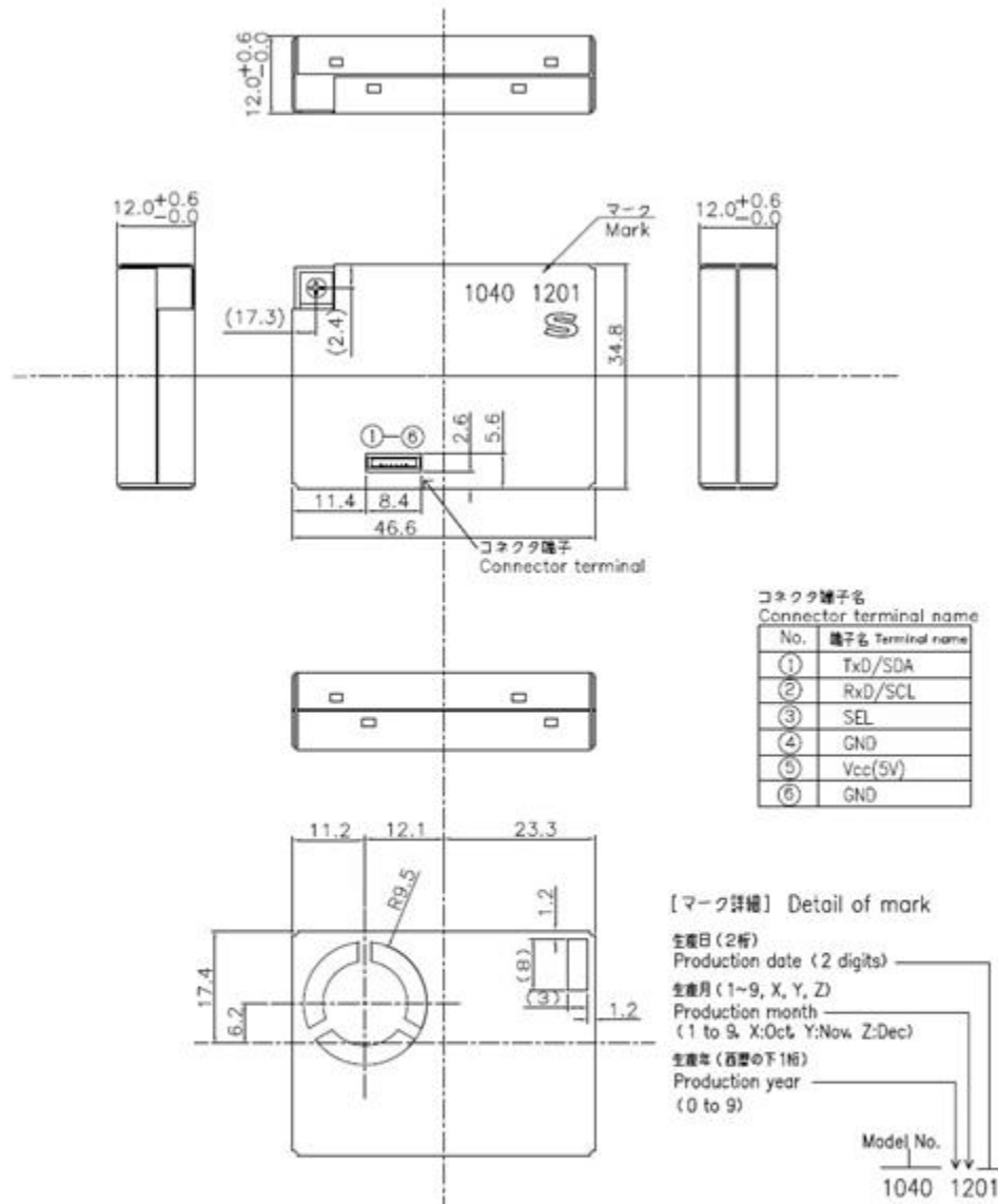
GP2Y1040AUF Outline Dimensions
