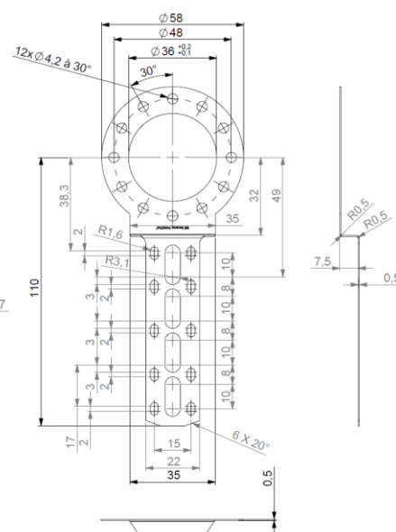
9445/047 tether arm
