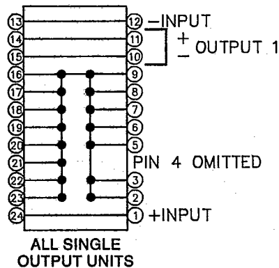
TOP VIEW VA
