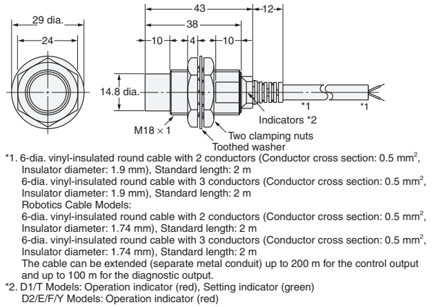
Diagram 11 E2E-X14MD□/E2E-X10ME□/F□ E2E-X10MY□
