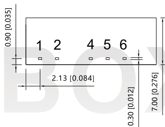
底视图
