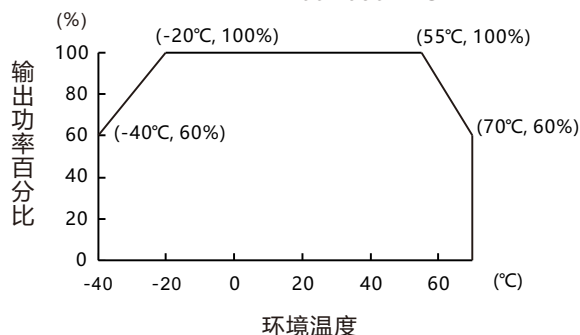
温度降额曲线 输入电压：85~465VAC 100~650VDC
