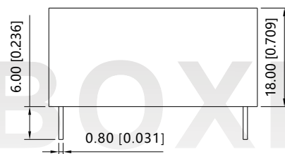
前视图
