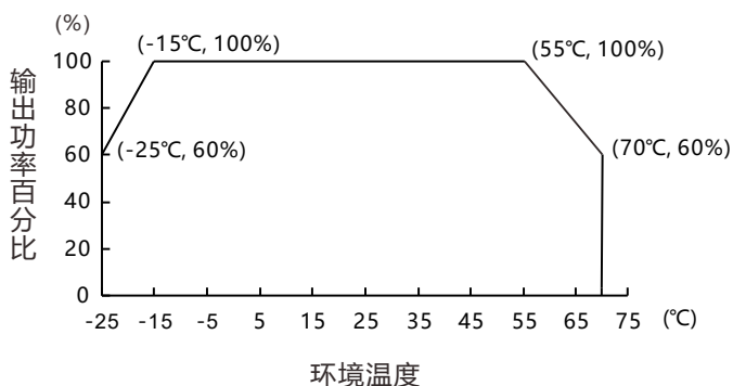
温度降额曲线 输入电压：85~264VAC 100~375VDC
