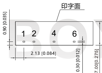
底视图
