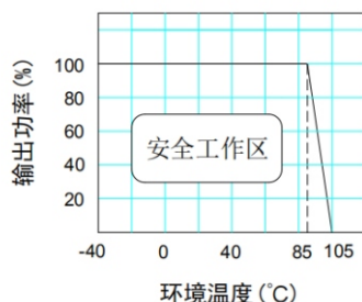
温度曲线图
