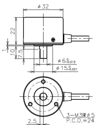
シャフトタイプ外形図
