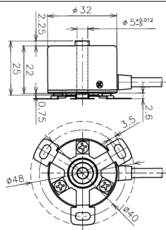
中空軸タイプ（貫通軸型）外形図
