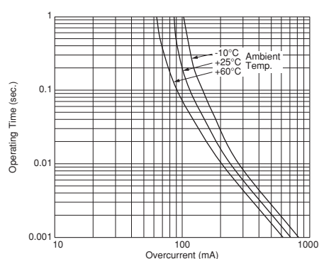
PRG15BC330MM1RC
