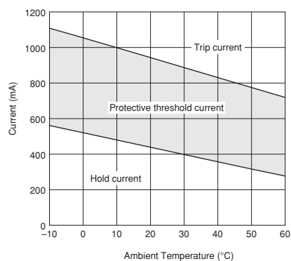
PRG21BC0R6MM1RA
