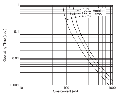
PRG15BC180MM1RC
