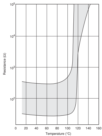
PTF_04BB222Q Type
