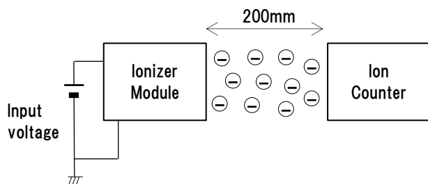
《 図 1-a 》イオン測定方法(イオンカウンター) 《 Fig.1-a 》Ion measurement(Ion counter)
