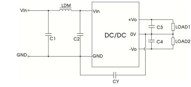
图 4.1 (其他输入推荐电路)
