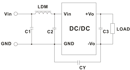
图 4.2 (5V 输入推荐电路)
