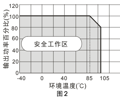
温度降额曲线图
