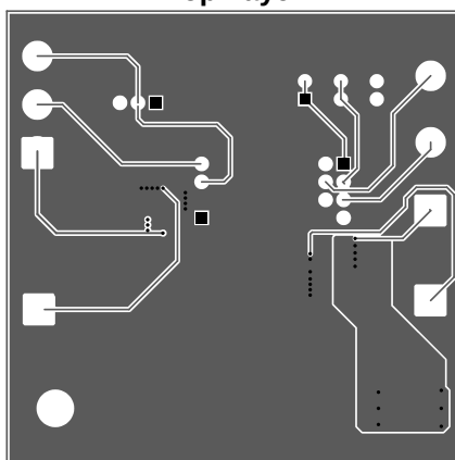
Mid Layer 2
