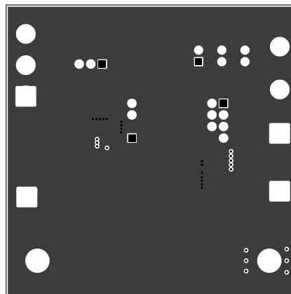
Mid Layer 1
