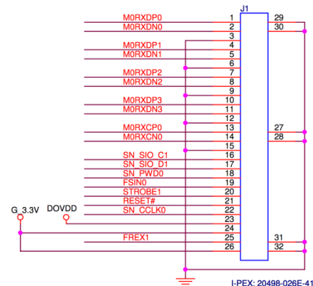
J1 (OV4689)
