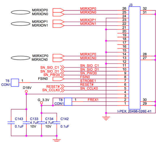
J3 (OV580)
