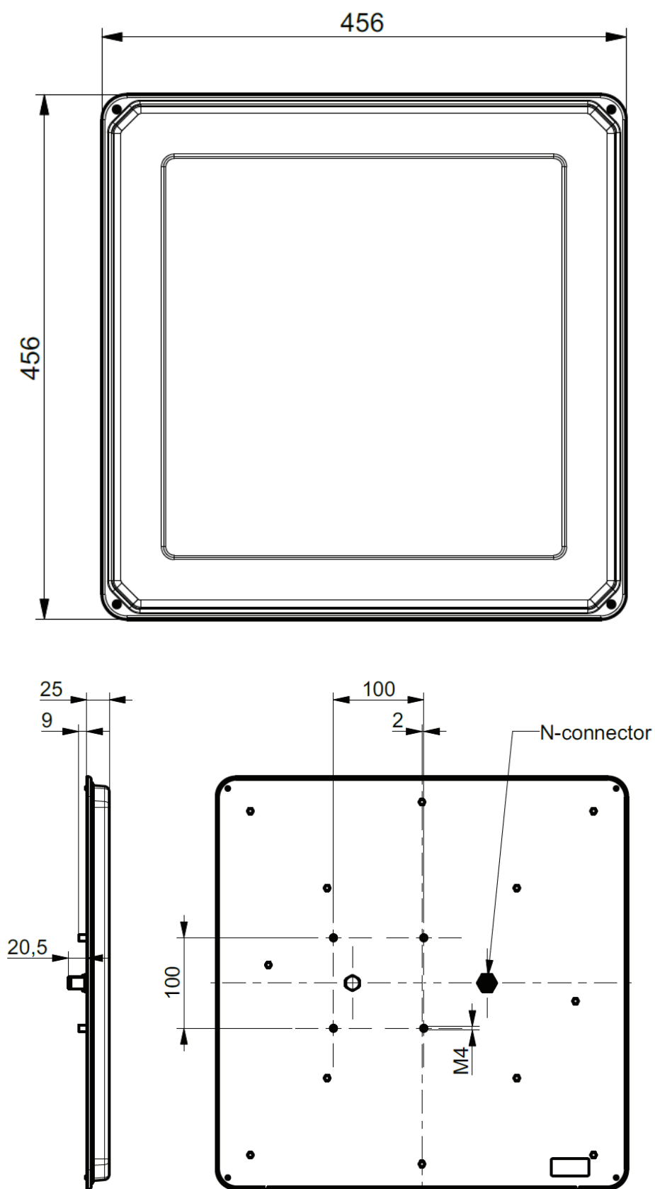
Bild 33: Abmessungen für WIRA 40° (52010251, -252)
