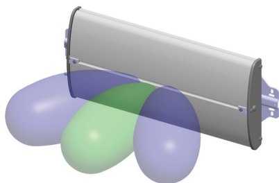
CSB antennas
