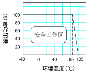
温度曲线图
