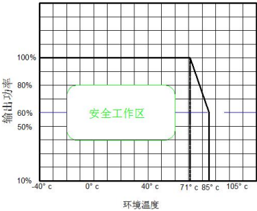
温度曲线图
