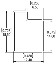
包装管尺寸图
