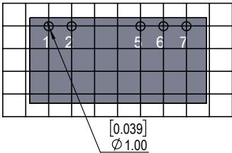
推荐 PCB 图 [0.1inch]2.54mm方格
