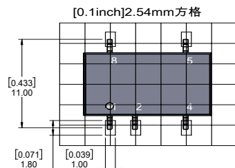
推荐 PCB 图
