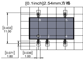
推荐 PCB 图
