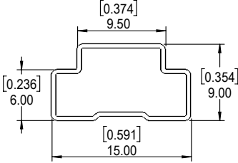
包装管尺寸图
