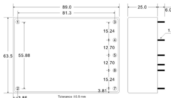
▲ ACE-M804A-R10 Dimensions
