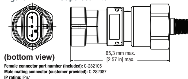
Figure 15. Deutsch 3-pin
