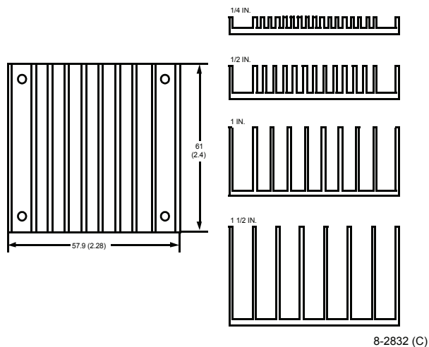
Figure 43. Longitudinal Heat Sink
