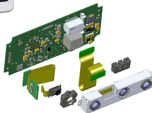
D435e module variant
