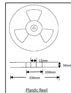
Fig. 10: Reel Dimensions
