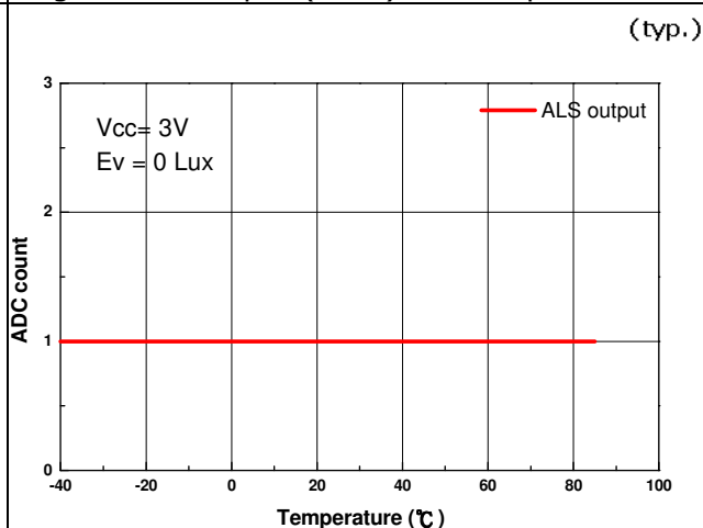
Fig.6 ALS output (Dark) vs. Temperature
