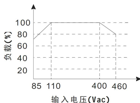
输入电压与负载曲线图
