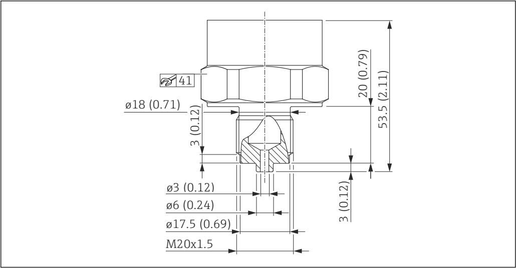
10 DIN 13 M20 x 1.5, EN 837, bore 3 mm (0.12 in)
