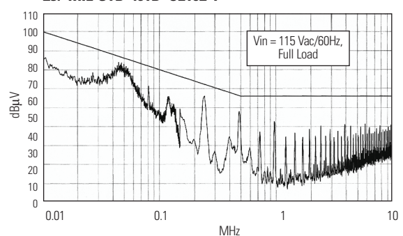
23. MIL-STD-461D CE102-1
