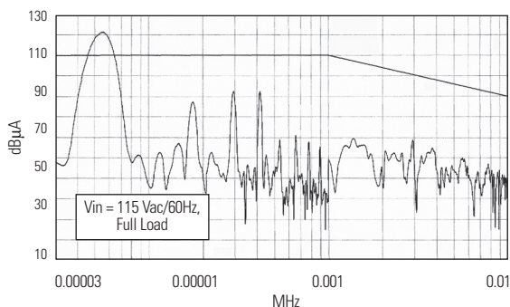
22. MIL-STD-461D CE101-4
