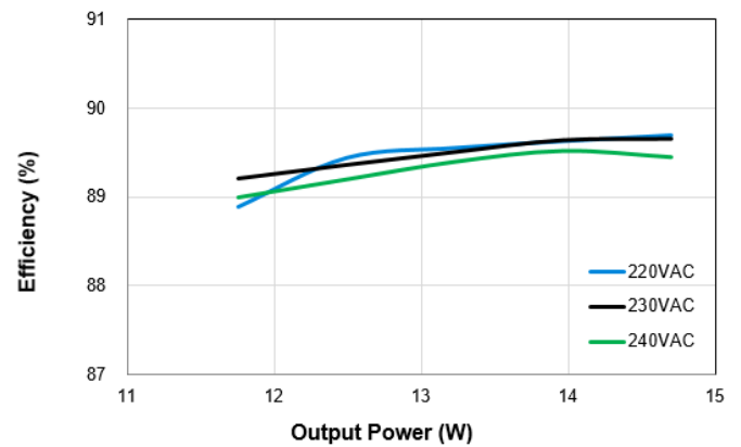
LNP-03A20WBCA – 350mA
