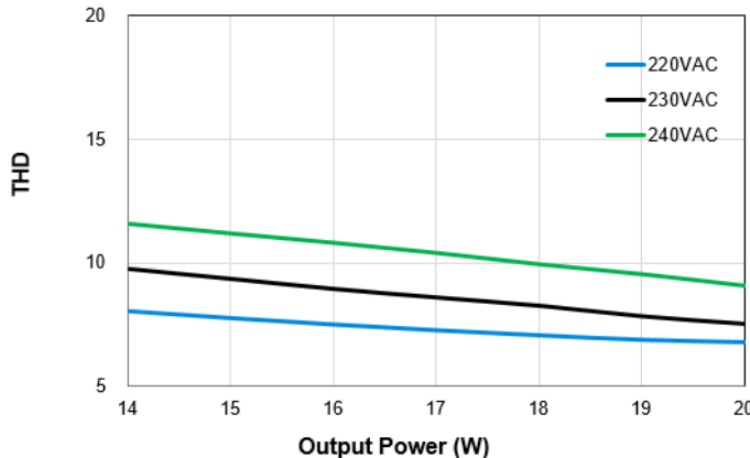
LNP-07A20WBCA – 700mA
