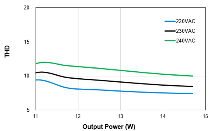
LNP-03A20WBCA – 350mA
