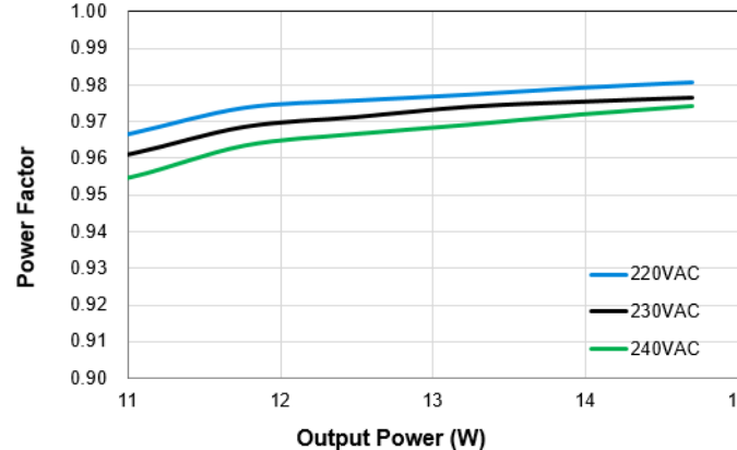
LNP-03A20WBCA – 350mA
