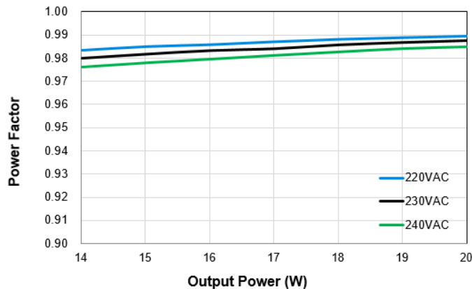
LNP-07A20WBCA – 700mA
