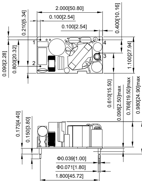
CFM25SXXX
