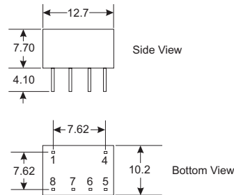
CTDD1210DF-TU1K-1 Package
