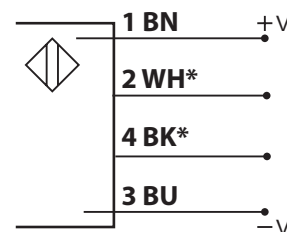
Fig. 6 Emitter
