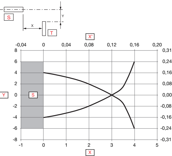
Fig. 4 Flush
