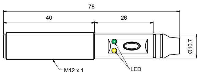
Fig. 6 Cable CA12CAF...A2IO
